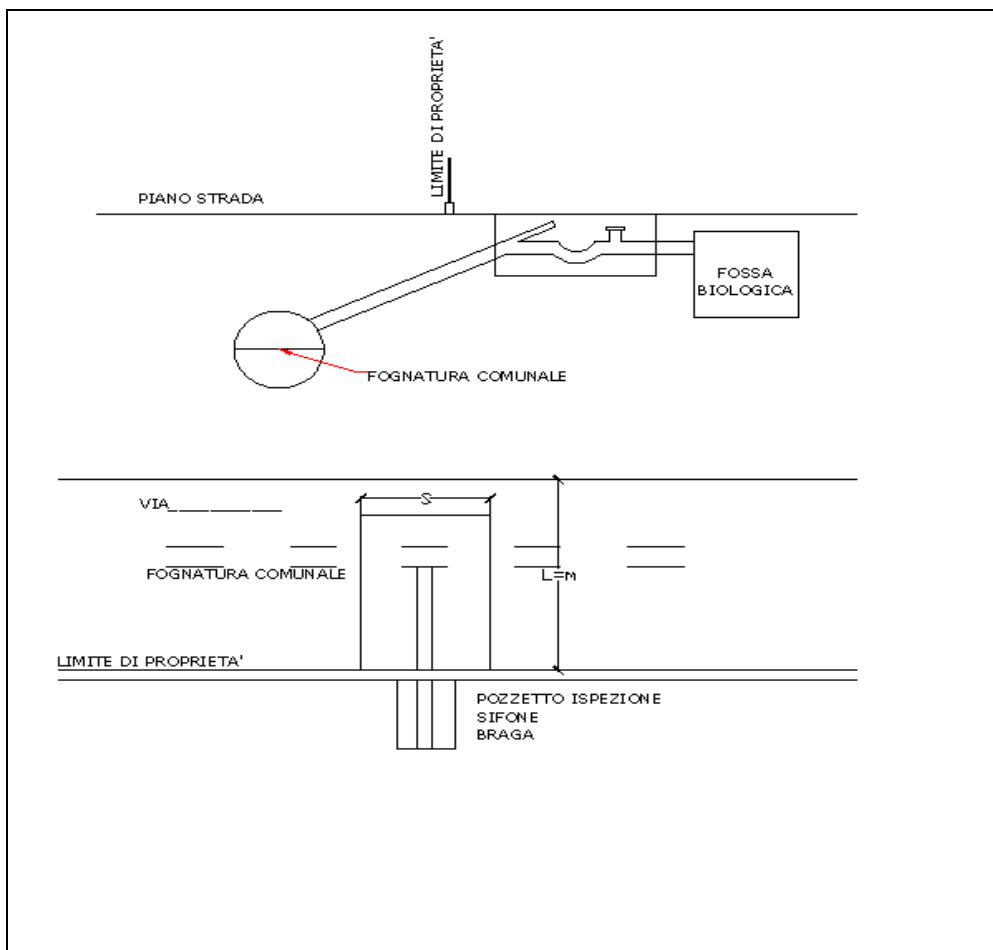
SEZIONE ALLACCIAMENTO RETE FOGNARIA COMUNALE E CALCOLO DEPOSITO CAUZIONALE PER MANOMISSIONE SUOLO PUBBLICO
